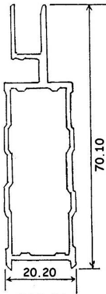
3575 0.707 KG/M
