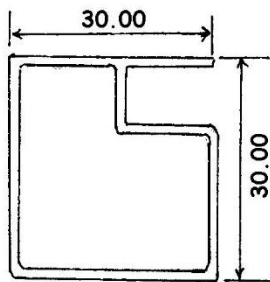
4174 0.437 KG/M
