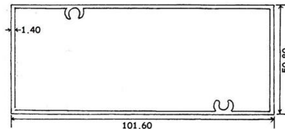
BX03182S 1.270 KG/M
