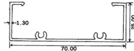
OP0321S 0.565 KG/M
