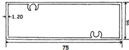
BX03102MS 0.72 KG/M
