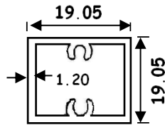
BX0303S 0.308 KG/M
