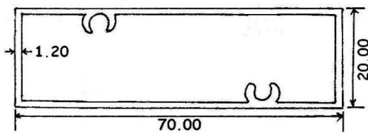
BX0325 0.671 KG/M
