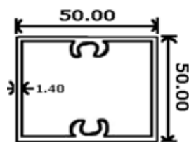
BX03062S 0.883 KG/M
