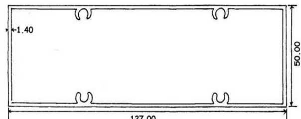
BX0333S 1.532 KG/M
