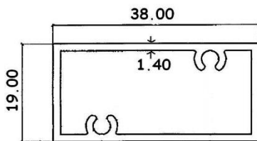
BX0334S 0.491 KG/M
