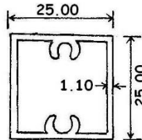
BX0304S 0.342 KG/M
