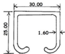
9205 0.393 KG/M
