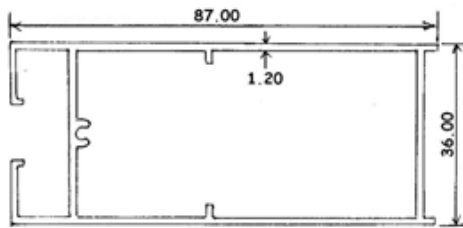
7801 1.037 KG/M
