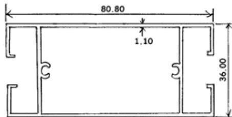
7802 0.845 KG/M
