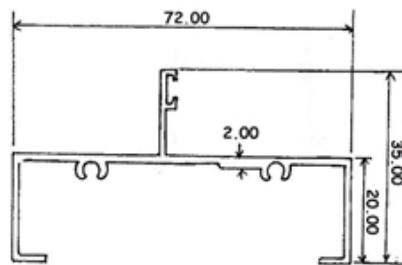
7804 0.566 KG/M
