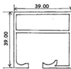
9201 0.721 KG/M
