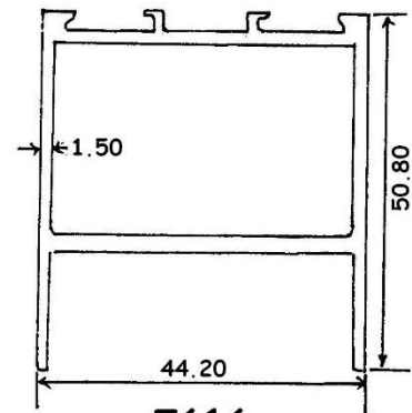
7616 0.909 KG/M
