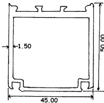
7620 0.927 KG/M
