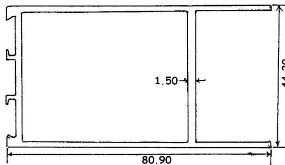
7615 1.154 KG/M
