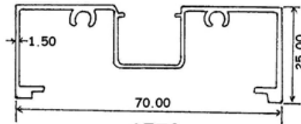
1578 0.679 KG/M
