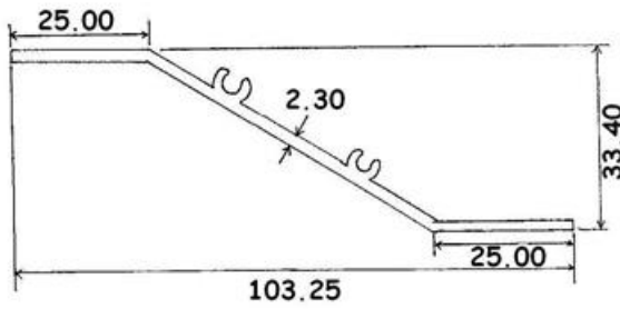
1571 0.813 KG/M
