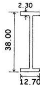
1570 0.383 KG/M
