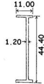
1568 0.208 KG/M
