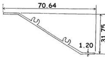
1563 0.321 KG/M
