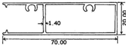
1583 0.772 KG/M
