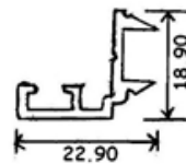
1581A 0.296 KG/M
