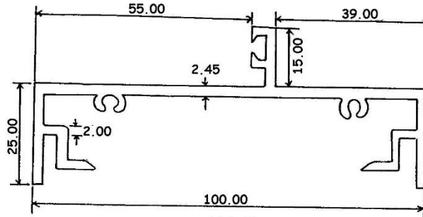
1574 1.463 KG/M
