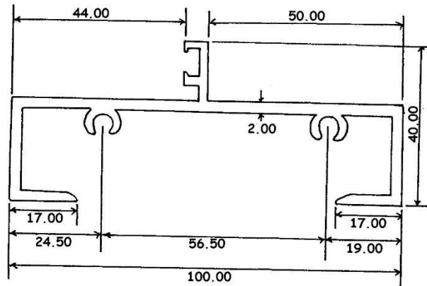
1573 1.216 KG/M
