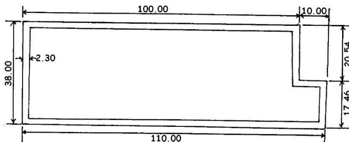
1576 1.870 KG/M
