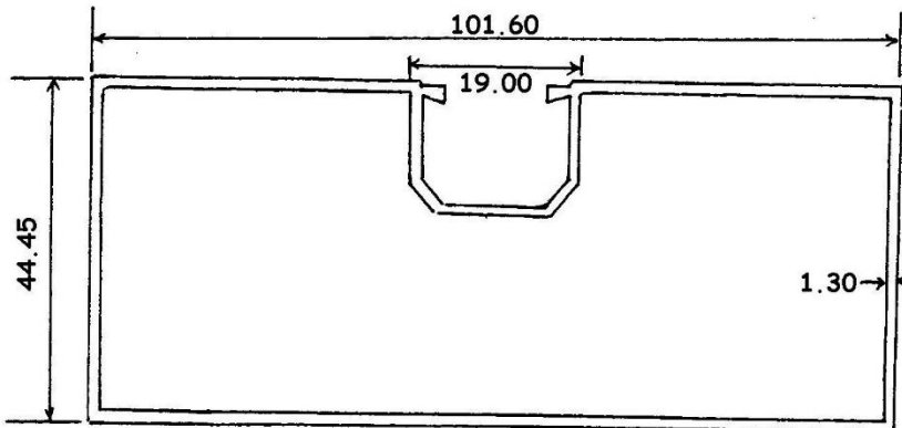
7507 1.138 KG/M
