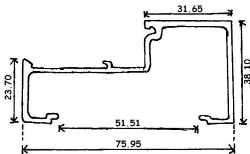
7305 0.682 KG/M
