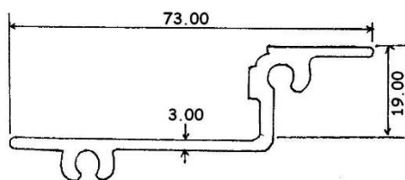
7300 0.886 KG/M
