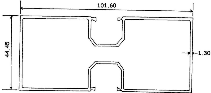
7508 1.263 KG/M
