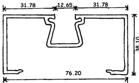
7306 0.793 KG/M
