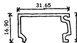
7303 0.238 KG/M
