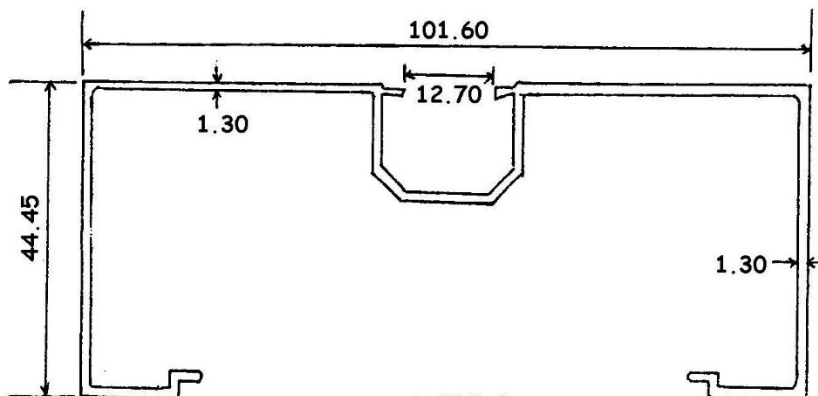
7506 0.905 KG/M
