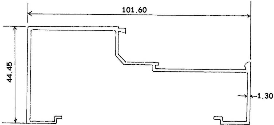
7505 0.826 KG/M
