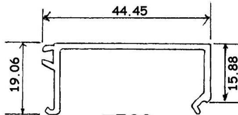
7503 0.341 KG/M
