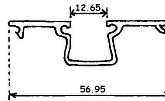
7302 0.359 KG/M
