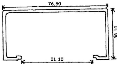
7304 0.597 KG/M
