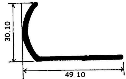
6109 0.292 KG/M
