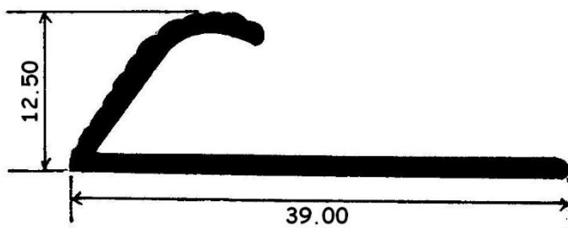
6108 0.189 KG/M
