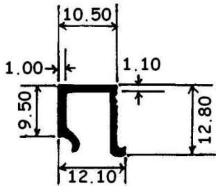
SPF 4 0.123 KG/M
