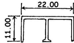
5300 0.149 KG/M
