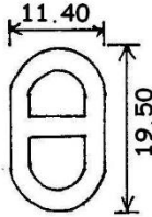
8449 0.26 KG/M
