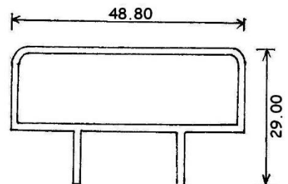
8116 0.372 KG/M
