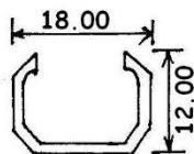
8339 0.102 KG/M
