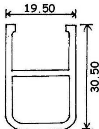
8225 0.239 KG/M
