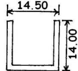
8337 0.099 KG/M
