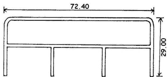
8111 0.614 KG/M
