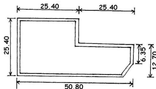
8422 0.399 KG/M
