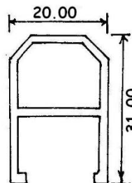
8229 0.267 KG/M
