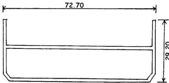
8119 0.530 KG/M
