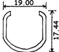
8333 0.116 KG/M
