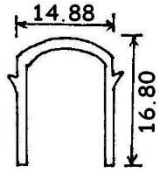
8334 0.11 KG/M
