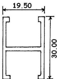
8227 0.213 KG/M
