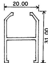
8230 0.247 KG/M
