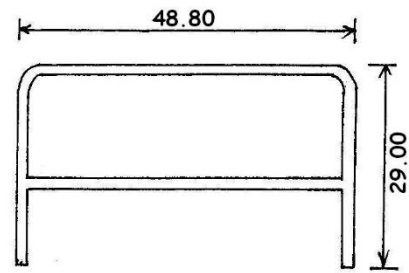
8117 0.369 KG/M
