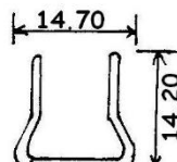
8338 0.112 KG/M
