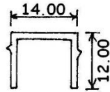
8336 0.09 KG/M
